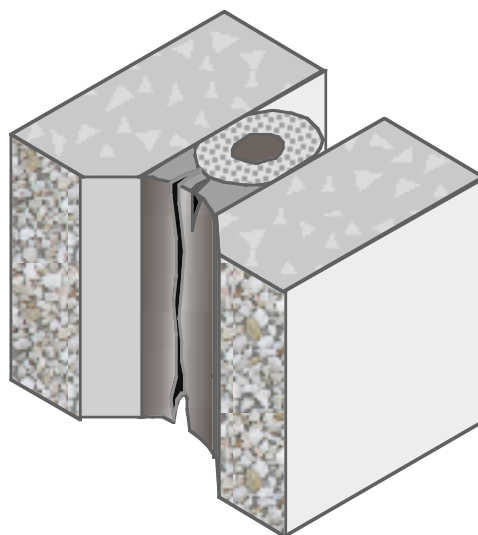
Figur 2. Sprickor i fogmassan (kohesionsbrott)
