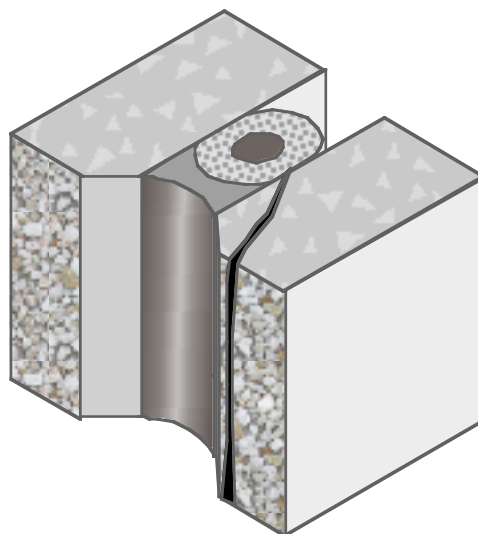
Figur 3. Avspjälkad fogsida
